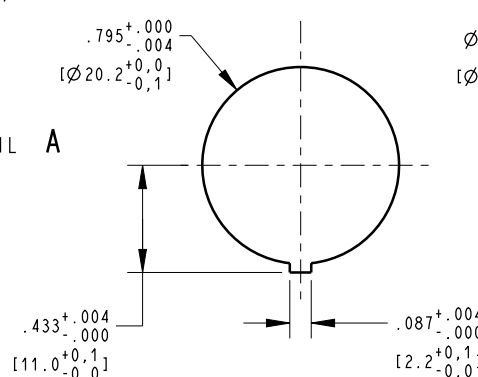
FIG. 1 SCALE 2:1
