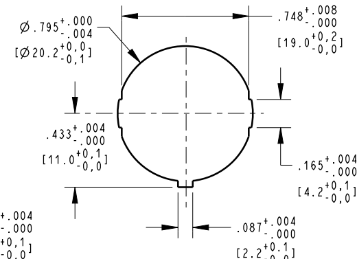
FIG. 2 SCALE 2:1
