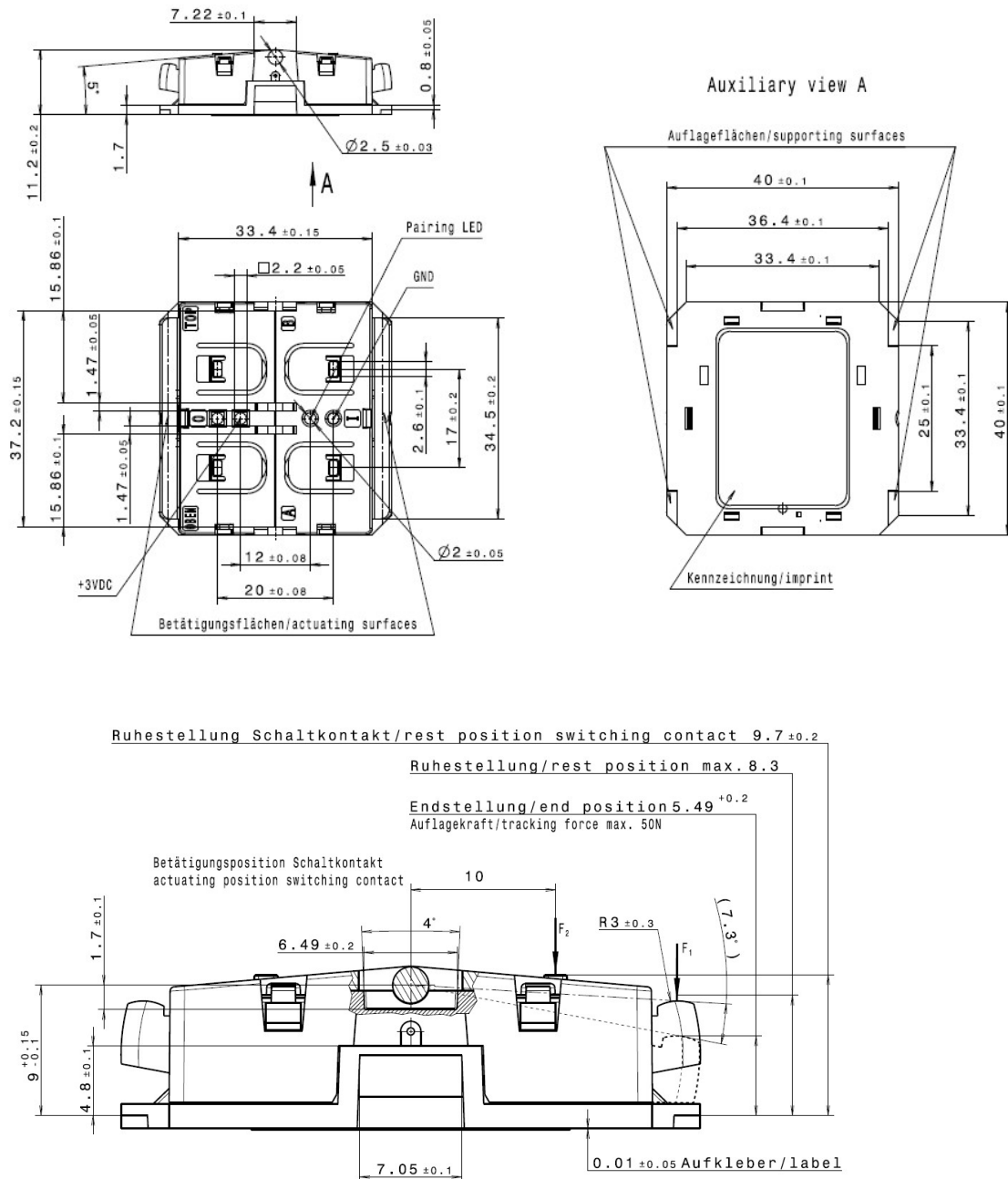
Bild / Picture 6 Abmessungen / Dimensions AFIM-1010
