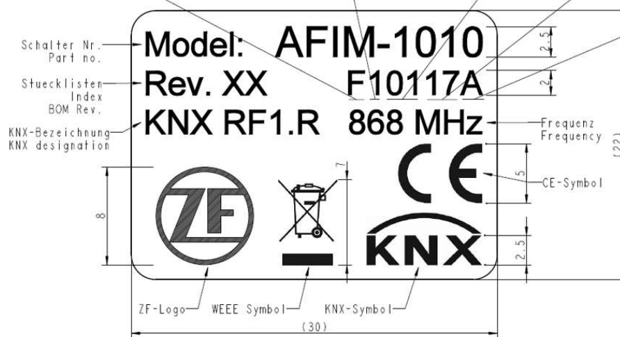
Bild / Picture 7 Aufkleber mit Inhalt zur Kennzeichnung / Label content
